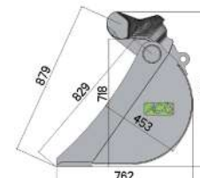
Profil P6N
