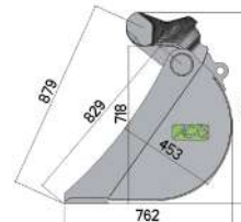
Profil P6N
