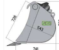
Profil PIN
