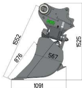
Profil 7IP1 2 x 45° - 2 Vérins
