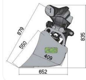
Profil 3IP1 2 x 45° - 1 Vérin
