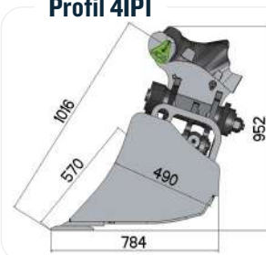
Profil 4IPI 2 x 45° - 2 Vérins
