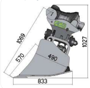
Profil 5IPI 2 x 45° - 2 Vérins
