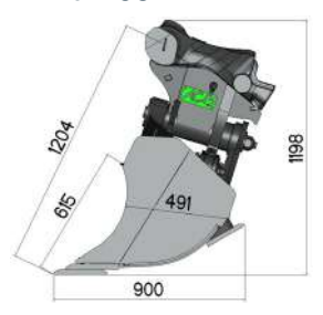
Profil 6CPI 2 x 45° - 2 Vérins
