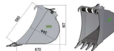
FEURST FK1TLR Épaisseur 20 mm
