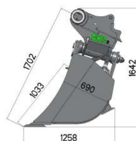
Profil 7IP2 2 x 45° - 2 Vérins
