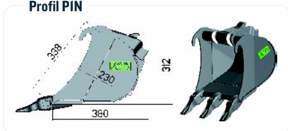
Profil PIN
