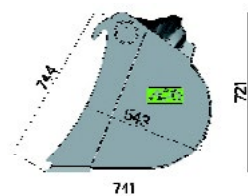
Profil P2N
