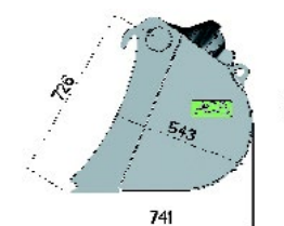
Profil PIN
